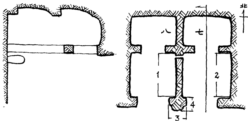
一、第七、八窟平面和第七窟剖面
